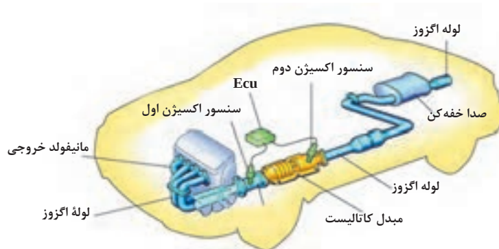
شکل ۲۰-۳ سیستم اگزوز برای موتور ردیفی
