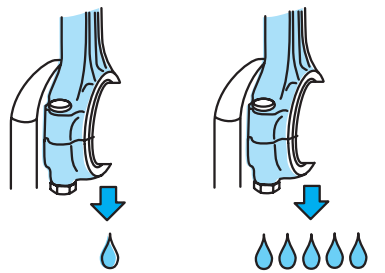
شکل ۹۵-۲ لقی دو برابر حد مجاز
