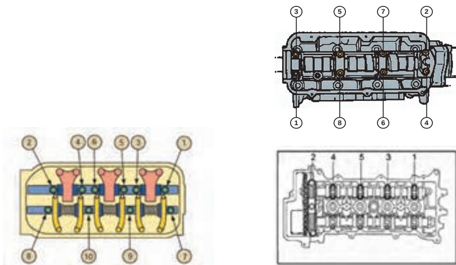
باز کردن پیچ‌های نگهدارنده میل اسبک
