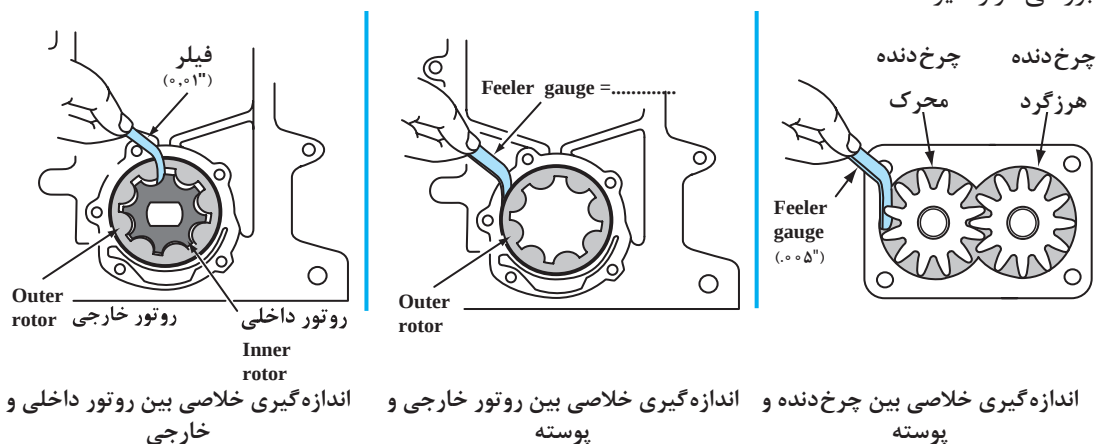
شکل ۲۸-۴ بررسی خوردگی و ساینده ای اجزای داخلی پمپ
