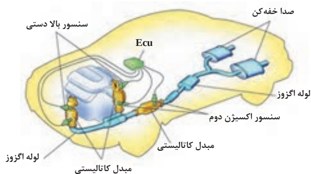
شکل ۱۹-۳ سیستم اگزوز برای خودرو با موتور V شکل
